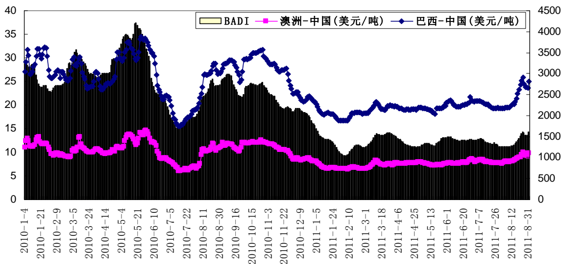
图 18: 国际铁矿石海运行情走势图
