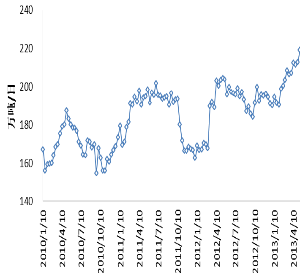
全国粗钢产量按旬统计
