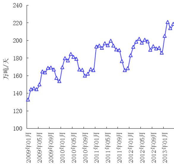
全国粗钢产量按月统计
